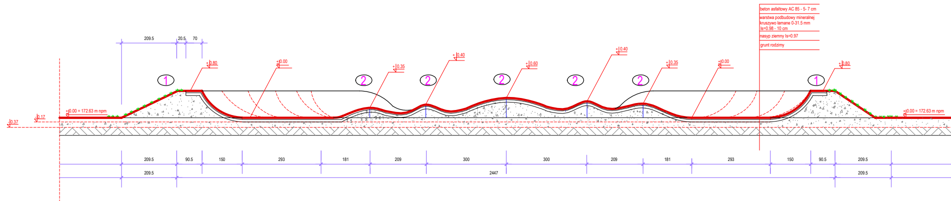
Przekrój A-A urządzeń toru PUMPTRACK
